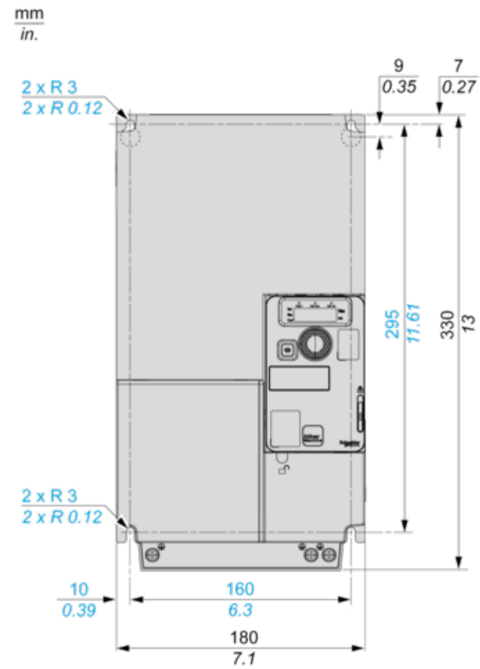
Vistas lateral derecha y frontal con placa CEM
