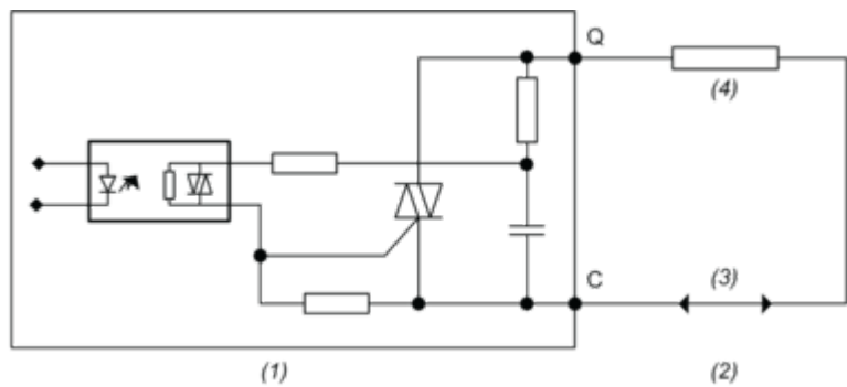
Diagrama del circuito de salida
